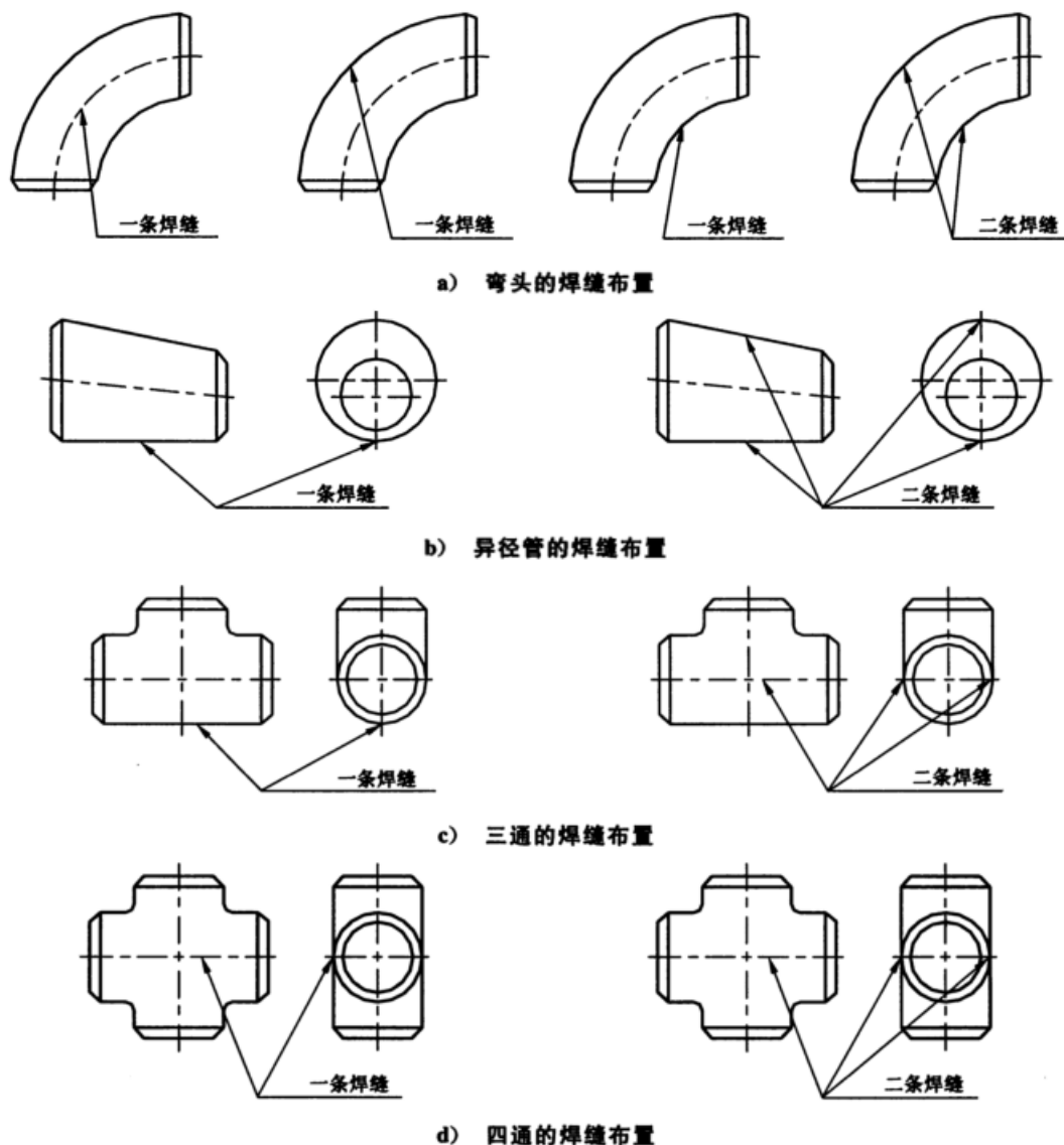
图 1 焊接管件的焊缝布置示意图
